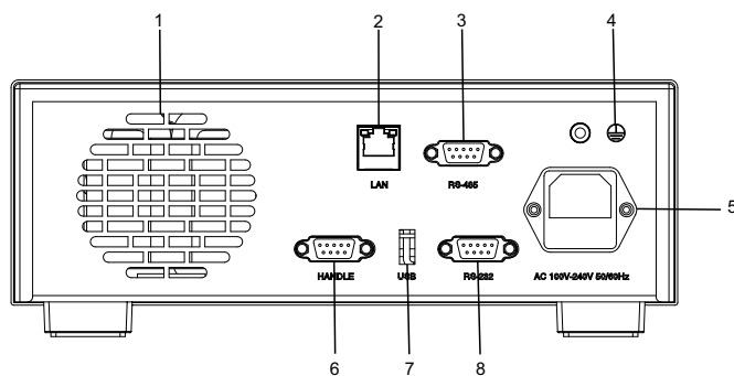
图 3-2 后面板说明
