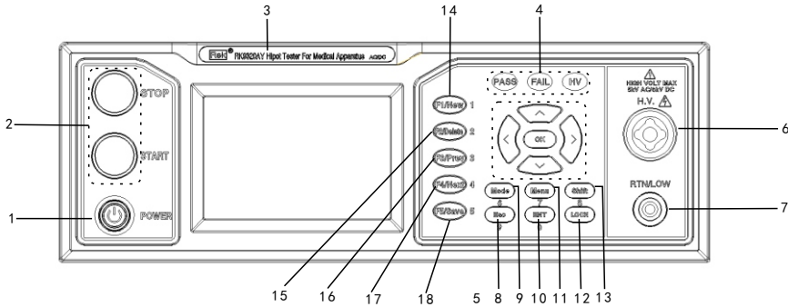
图 3-1 对 RK93XX 系列前面板进行了简要说明。
