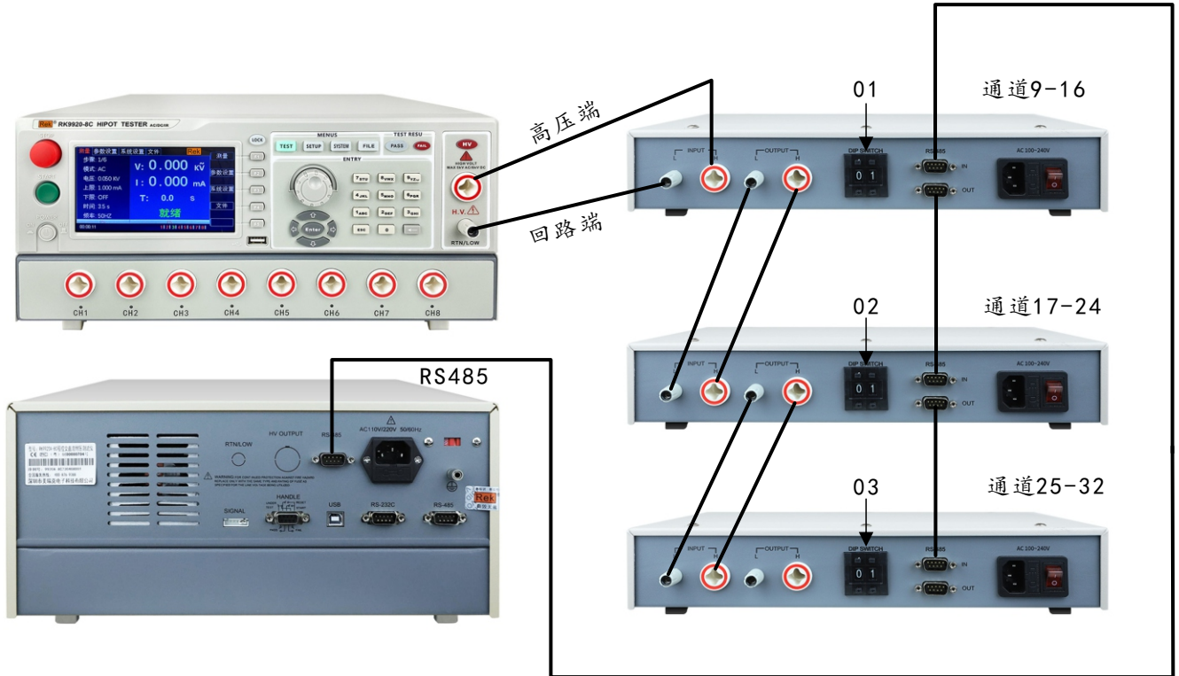
RK9920-8C主机与RK-8CH串行扫描盒通讯连接
