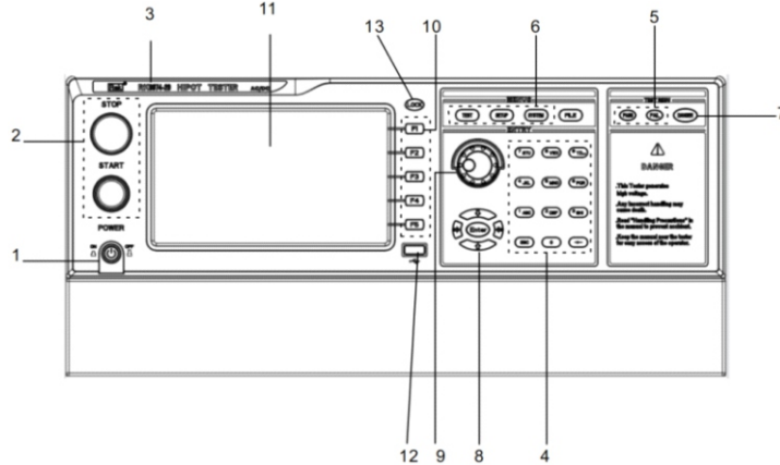
图 3-1 前面板说明
