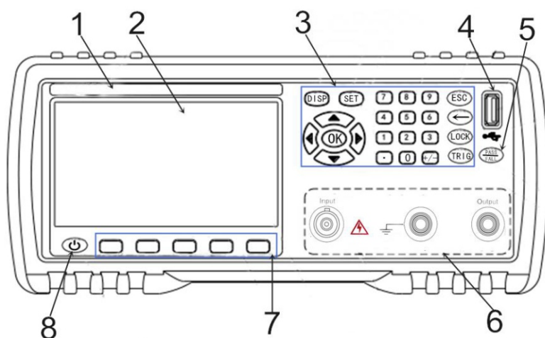
图2-1 前面板
